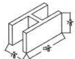
Double Endout
